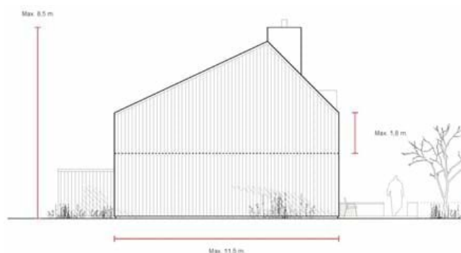
Eksempel på udformning af byggeri i 2 etager med trappe
