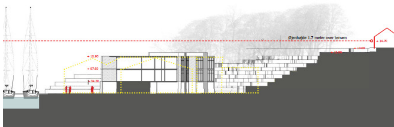
Tværsnit gennem ny boligbebyggelse fra lystbådehavn, kaj anlæg, bagvedliggende kystskrånning, ny bebyggelse med parkering i stueniveau og boliglejligheder på 1. og 2. etage, kystskrånning og privat have med terrasse og parcelhus.
