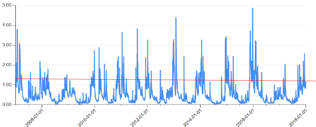
Figur 2: Målte vandføringer (m 3 /s) i Hundstrup Å ved st. 6.86 m ved Elleskov Mølle i perioden fra 2008 til 2018. Den røde streg viser den omtrentlige placering af vandføringen på 1.295 l/s over den målte 10 årige periode.
