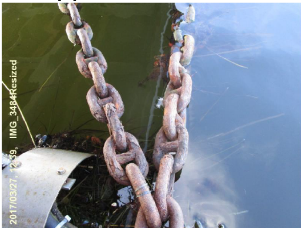
Eksempel på korrosion af forankringskæder.
