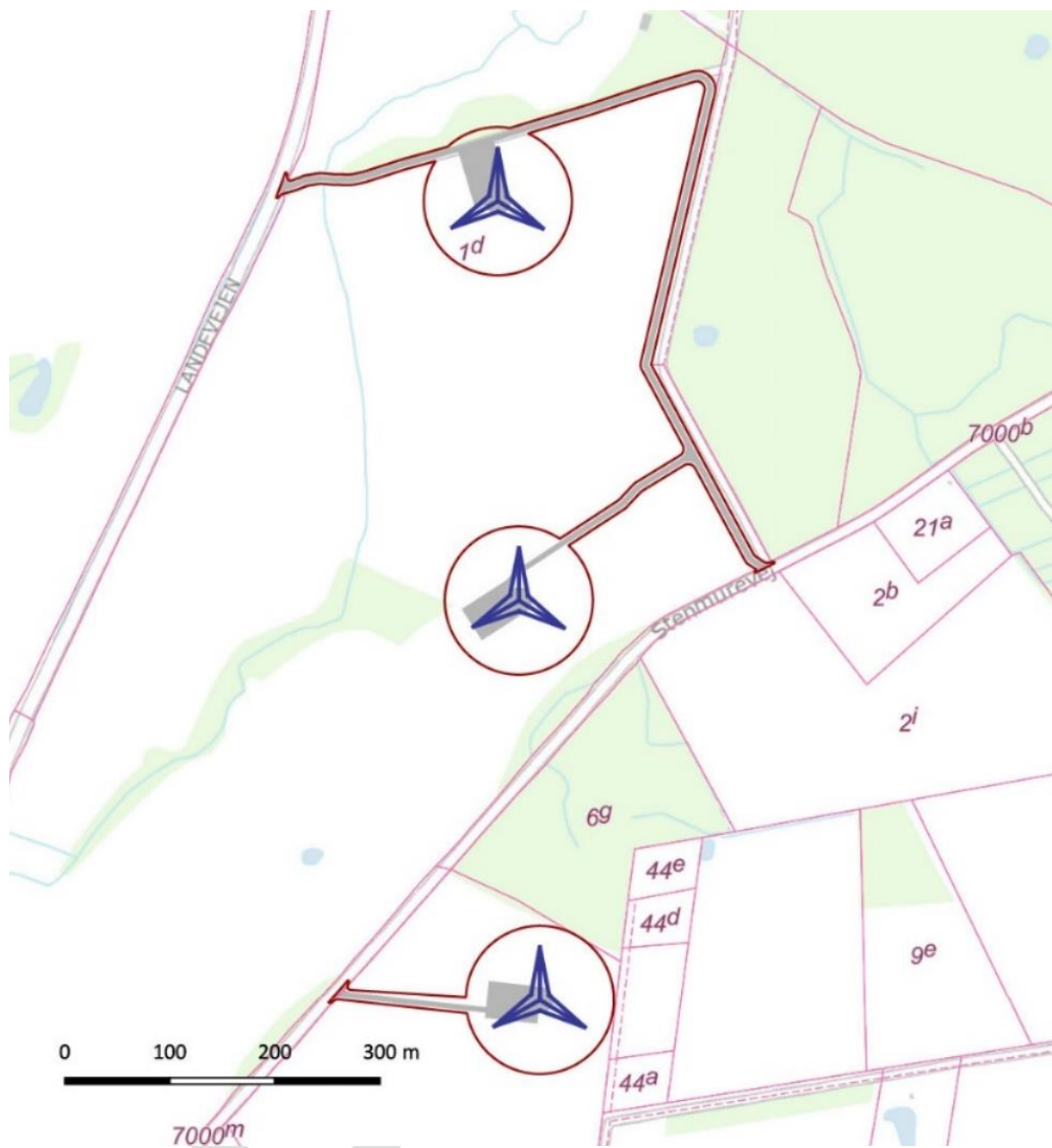
Figur 1 - Lokalplanens afgrænsning og placering af vindmøller, adgangsveje og servicepladser.
