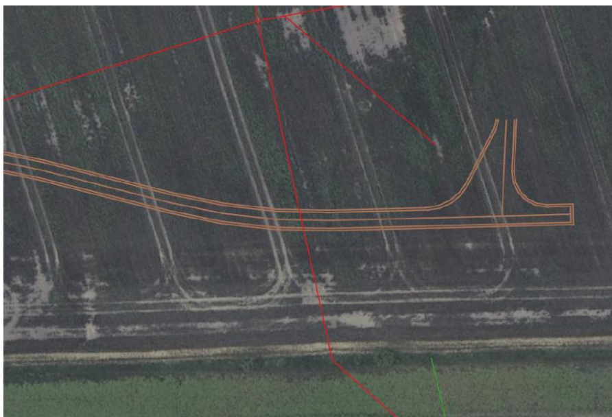
Figur 2: Nord-sydgående rød streg angiver eksisterende rørlagt vandløb. Forsyningsvej er angivet med brune streger. Ny rørunderføring etableres, hvor de to krydser hinanden. Målestoksforhold 1:1000.
