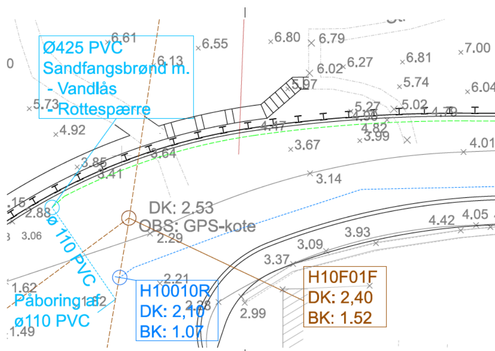
Figur 2: Oversigt over drænlednings (markeret med grønt)
