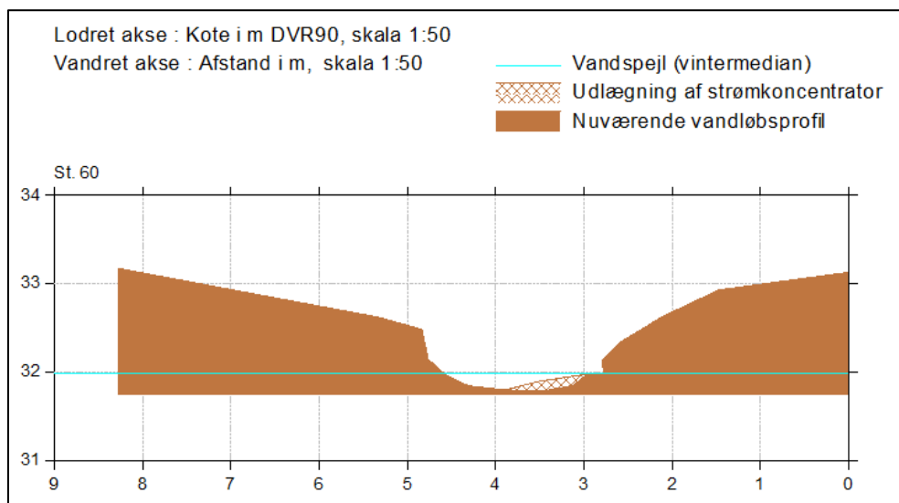
Figur 5: Udlægning af strømkoncentrator i st. 60 m.
