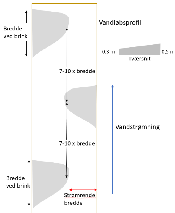
Figur 3: Principskitse for udlægning af strømkoncentratorer.
