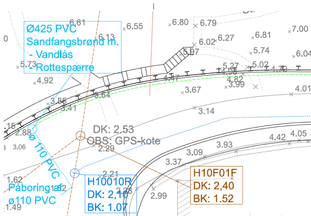
Figur 2: Oversigt over planlagt placering af drænledning (markeret med grønt)
