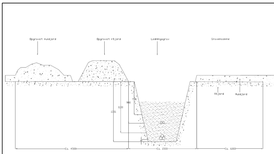
Figur 3: Graveprofil
